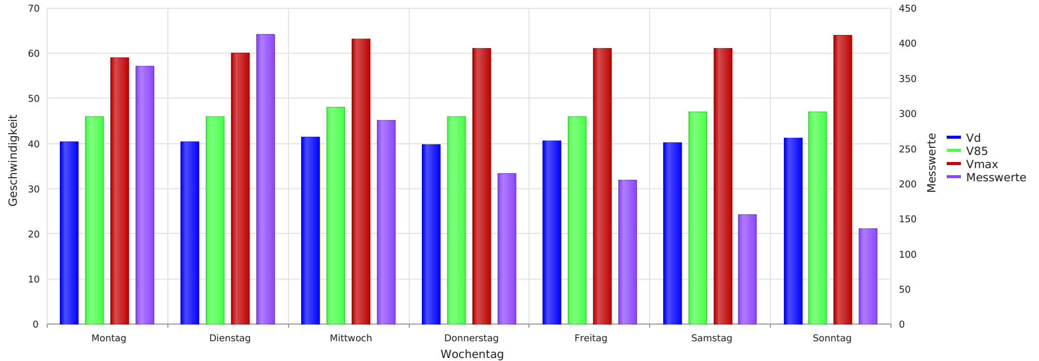
Ferenbalm - Ferenbalmstrasse 30, FR Biberen, 40 kmh Beschränkung Vd, V85, Vmax, Anzahl der Messwerte vs. Wochentag
