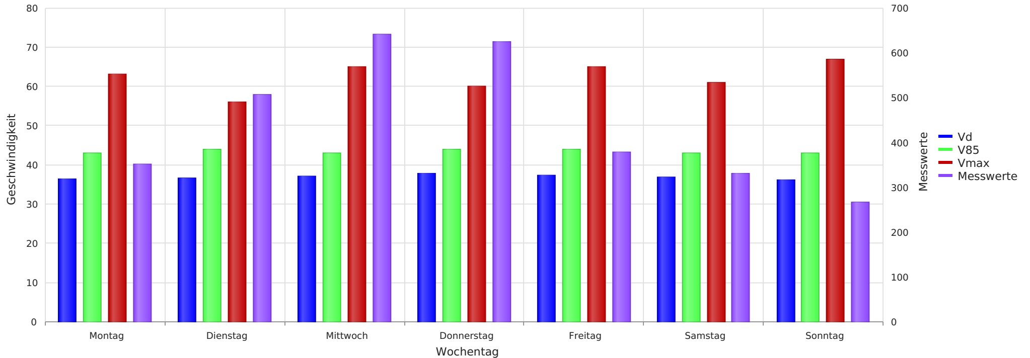
Rizenbach, Längacker 7, Fahrtrichtung Gümmenen, 40 km/h Beschränkung Vd, V85, Vmax, Anzahl der Messwerte vs. Wochentag
