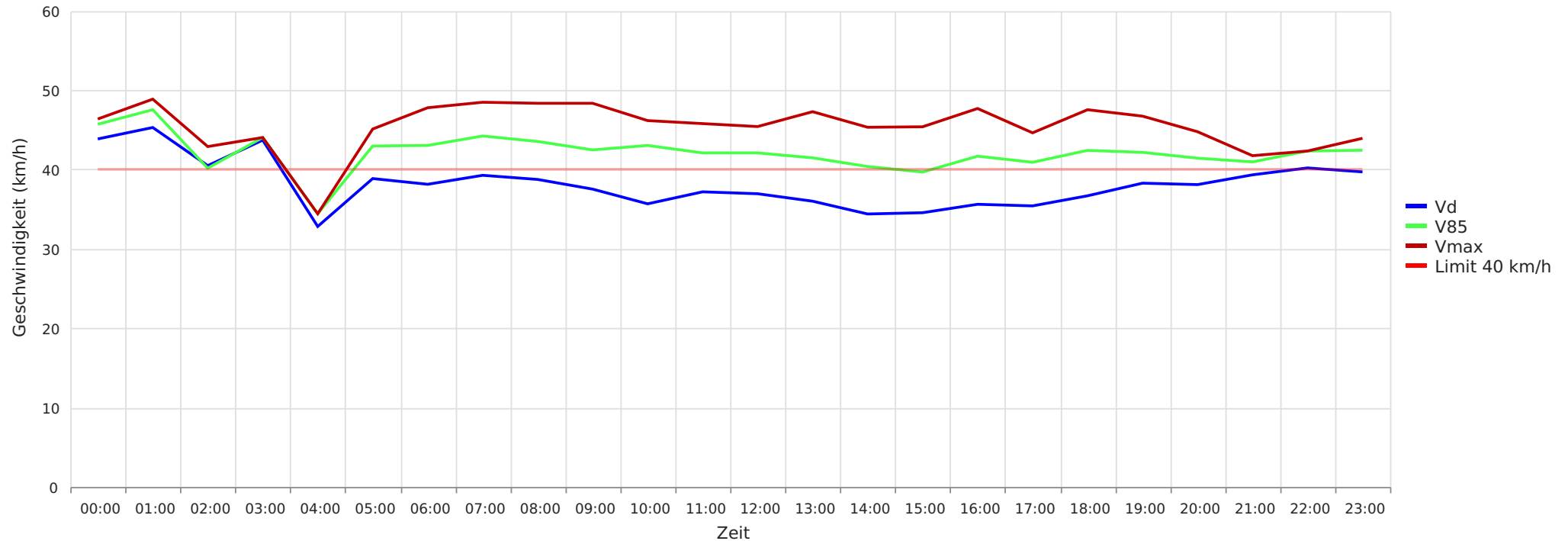
Rizenbach, Längacker 7, Fahrtrichtung Gümmenen, 40 km/h Beschränkung Vd, V85, Vmax vs. Uhrzeit
