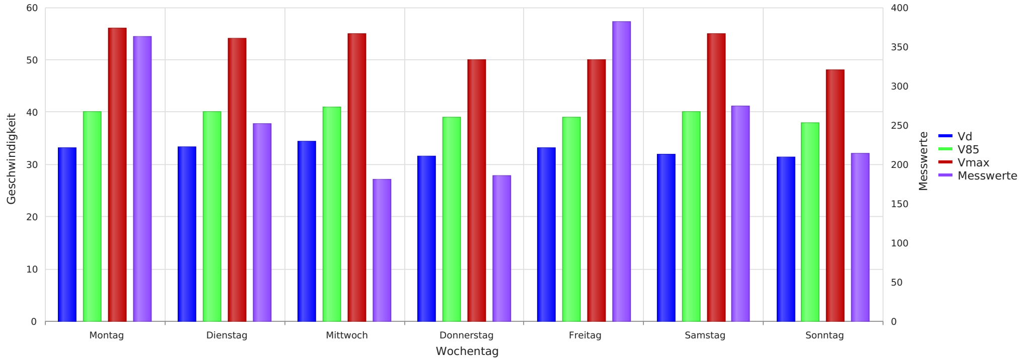
Strasse Rizenbach - Längacker 11, Fahrtrichtung Biberen, 40 km/h Beschränkung Vd, V85, Vmax, Anzahl der Messwerte vs. Wochentag
