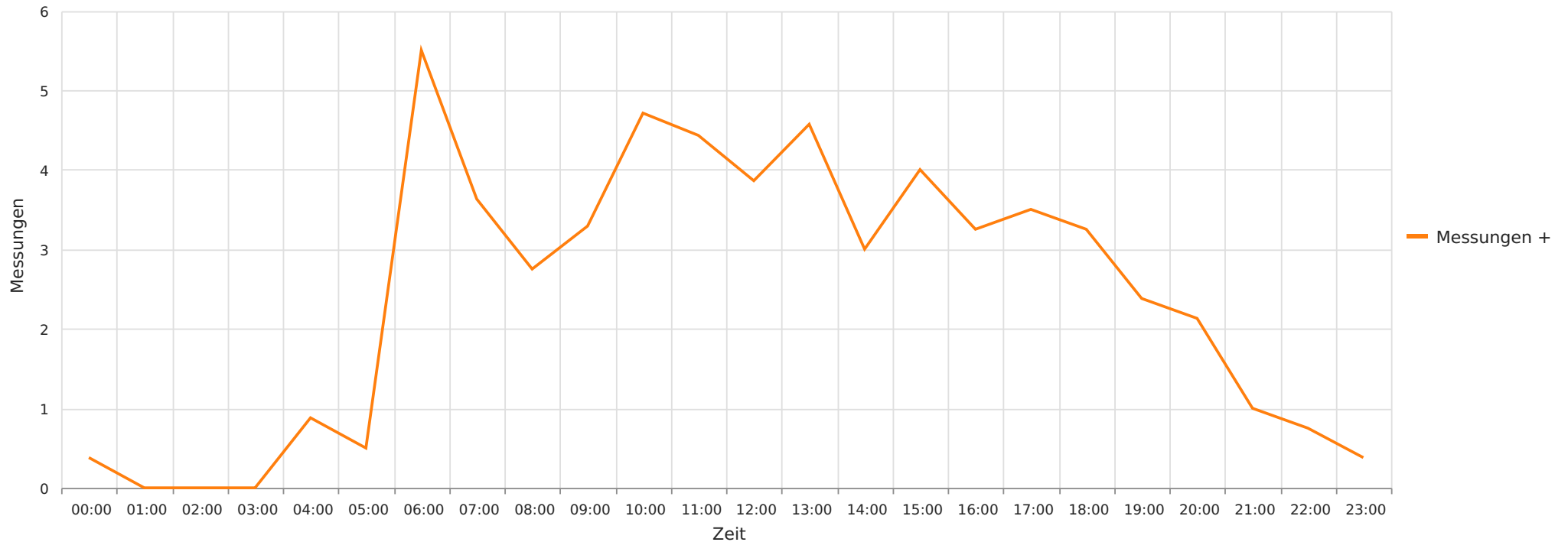
Gümmenen - Wittenberg 16, Fahrtrichtung Wittenberg, 50 km/h Beschränkung Gemittelte Anzahl an Messwerten vs. Uhrzeit
