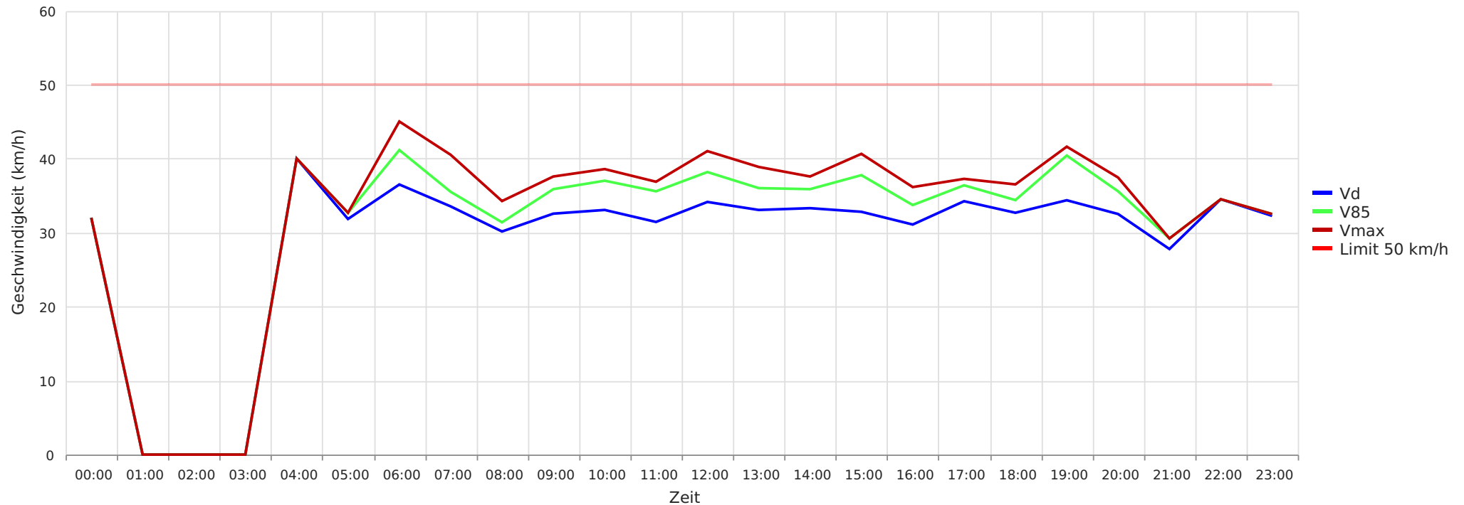
Gümmenen - Wittenberg 16, Fahrtrichtung Wittenberg, 50 km/h Beschränkung Vd, V85, Vmax vs. Uhrzeit
