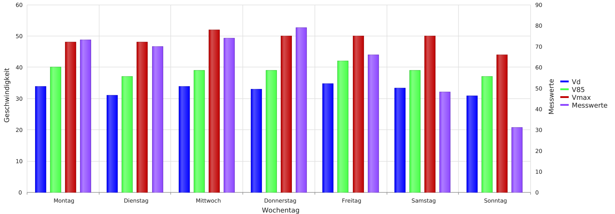
Gümmenen - Wittenberg 16, Fahrtrichtung Wittenberg, 50 km/h Beschränkung Vd, V85, Vmax, Anzahl der Messwerte vs. Wochentag
