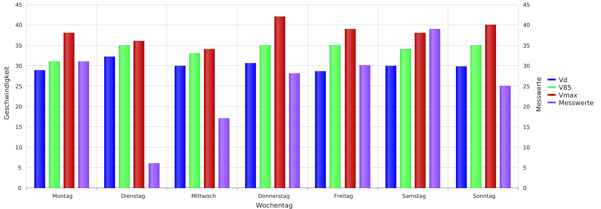
Gümmenen - Wittenberg 16, Fahrtrichtung Bahnhof, 50 km/h Beschränkung Vd, V85, Vmax, Anzahl der Messwerte vs. Wochentag
