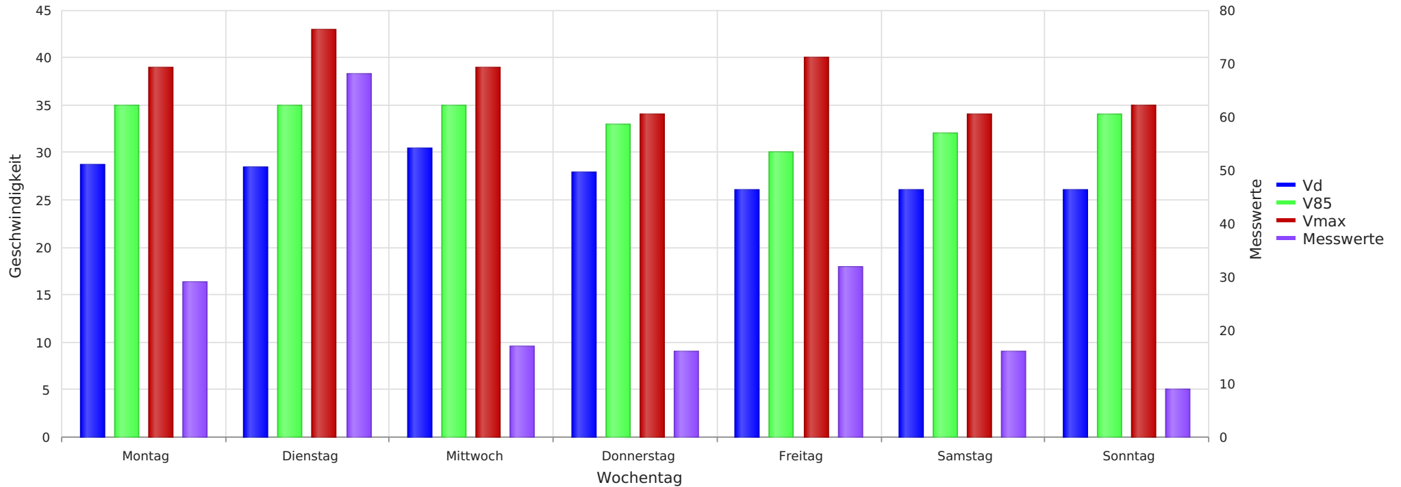
Biberen - Unterdorfstrasse 4, Fahrtrichtung Hemtech, 50 km/h Beschränkung Vd, V85, Vmax, Anzahl der Messwerte vs. Wochentag
