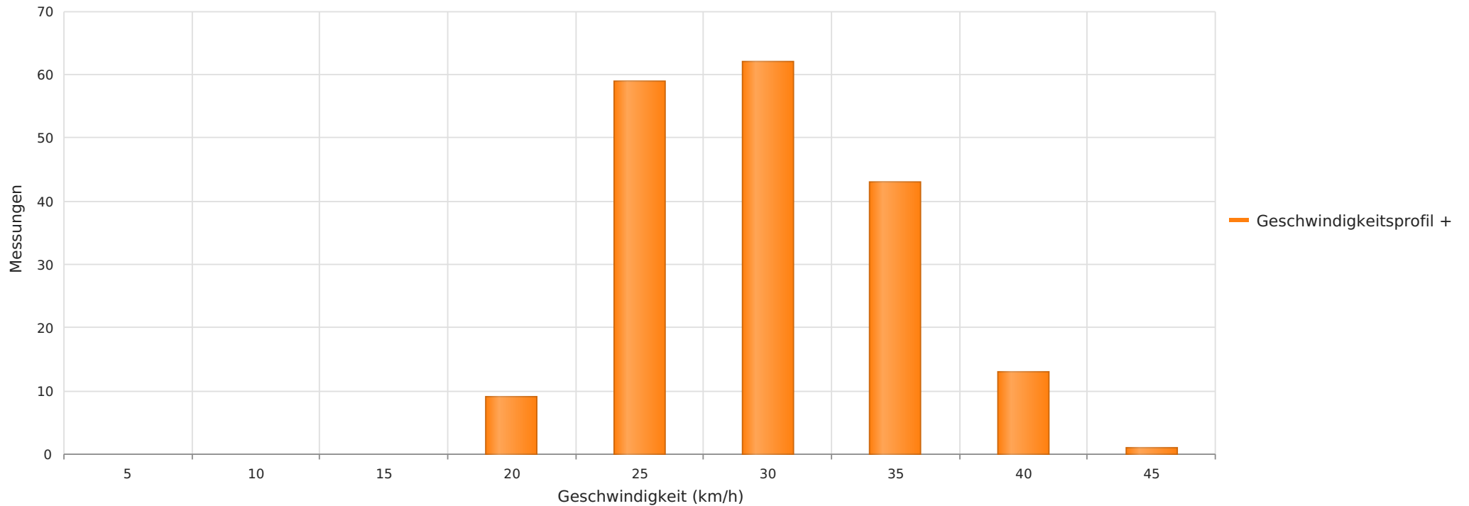
Biberen - Unterdorfstrasse 4, Fahrtrichtung Hemtech, 50 km/h Beschränkung Anzahl der Messwerte vs. Geschwindigkeit
