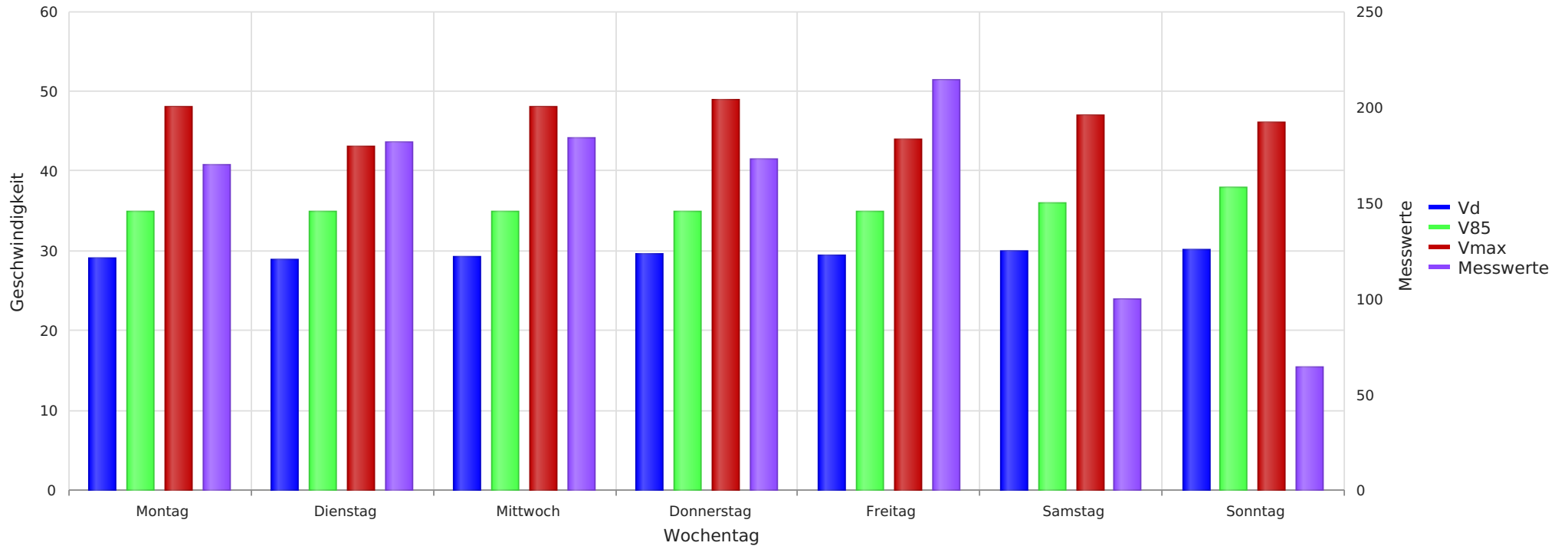
Biberen - Unterdorfstrasse 4, Fahrtrichtung Rytz, 50 km/h Beschränkung Vd, V85, Vmax, Anzahl der Messwerte vs. Wochentag
