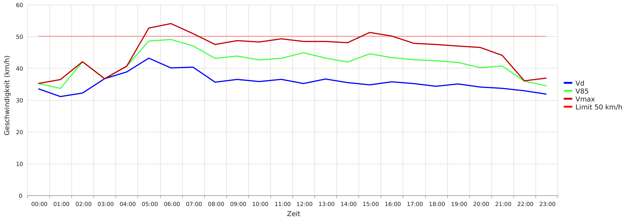
Gammen - Dorfstrasse 18B, Fahrtrichtung Altes Schulhaus, 50 km/h Beschränkung Vd, V85, Vmax vs. Uhrzeit
