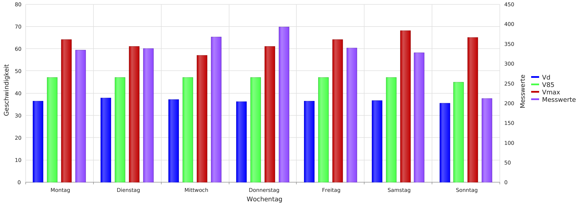
Gammen - Dorfstrasse 18B, Fahrtrichtung Altes Schulhaus, 50 km/h Beschränkung Vd, V85, Vmax, Anzahl der Messwerte vs. Wochentag
