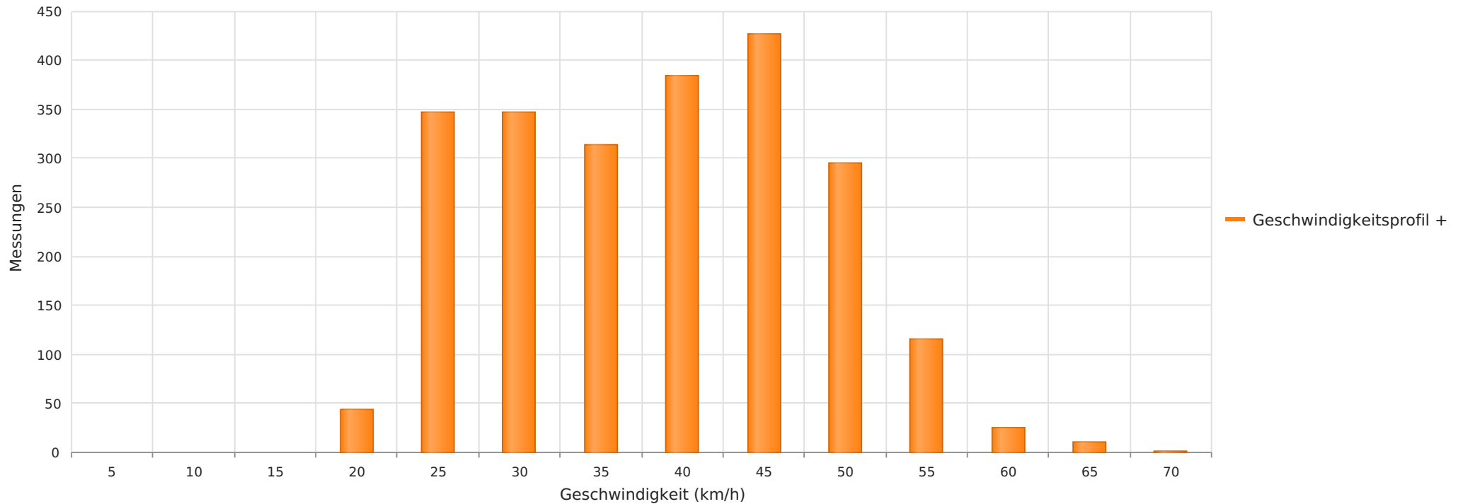
Gammen - Dorfstrasse 18B, Fahrtrichtung Altes Schulhaus, 50 km/h Beschränkung Anzahl der Messwerte vs. Geschwindigkeit
