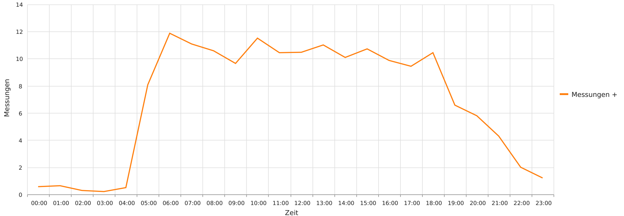
Gammen - Dorfstrasse 18B, Fahrtrichtung Altes Schulhaus, 50 km/h Beschränkung Gemittelte Anzahl an Messwerten vs. Uhrzeit
