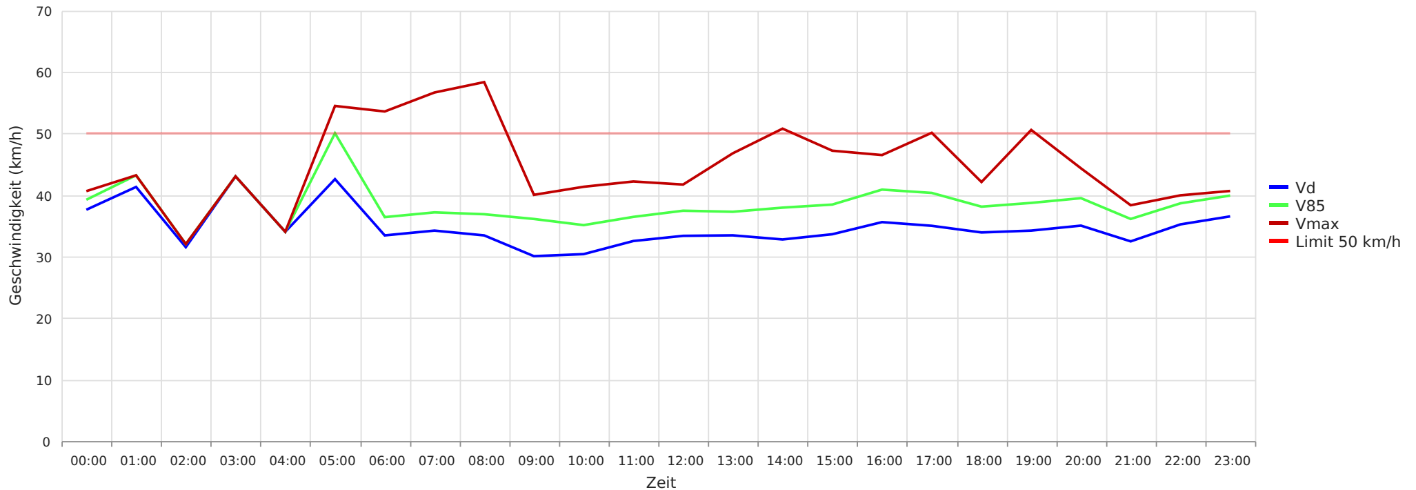
Gammen - Dorfstrasse 18B, Fahrtrichtung Biberen, 50 km/h Beschränkung Vd, V85, Vmax vs. Uhrzeit
