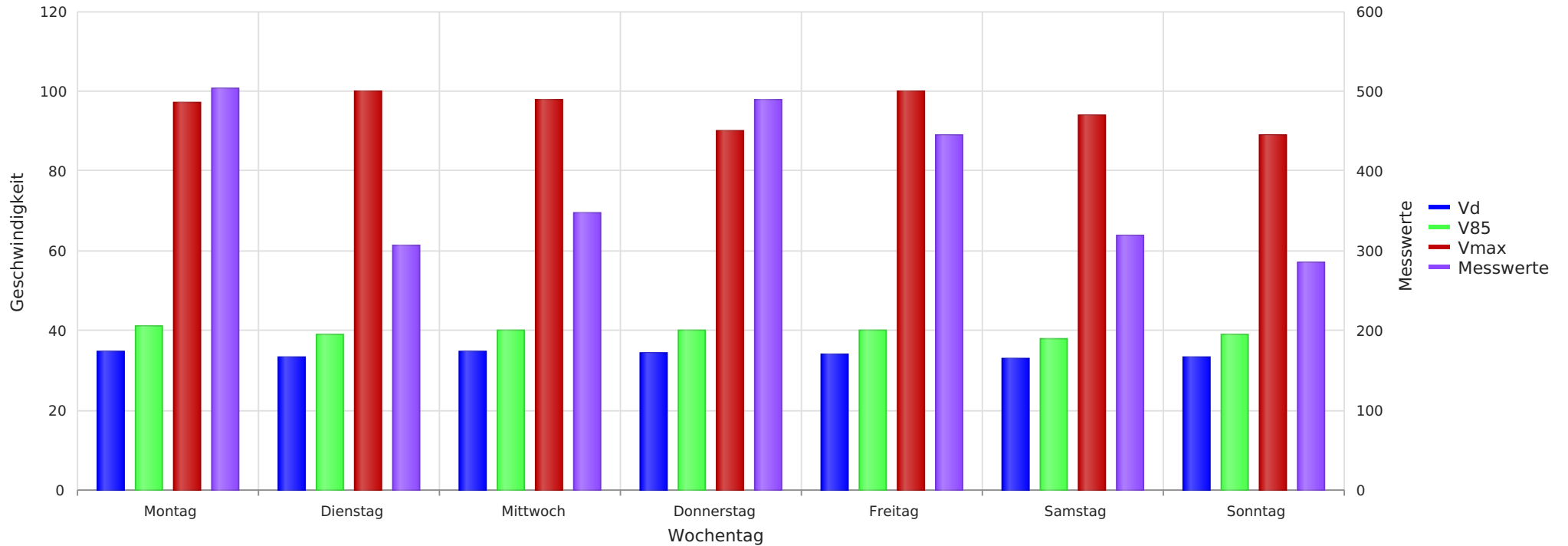
Gammen - Dorfstrasse 18B, Fahrtrichtung Biberen, 50 km/h Beschränkung Vd, V85, Vmax, Anzahl der Messwerte vs. Wochentag
