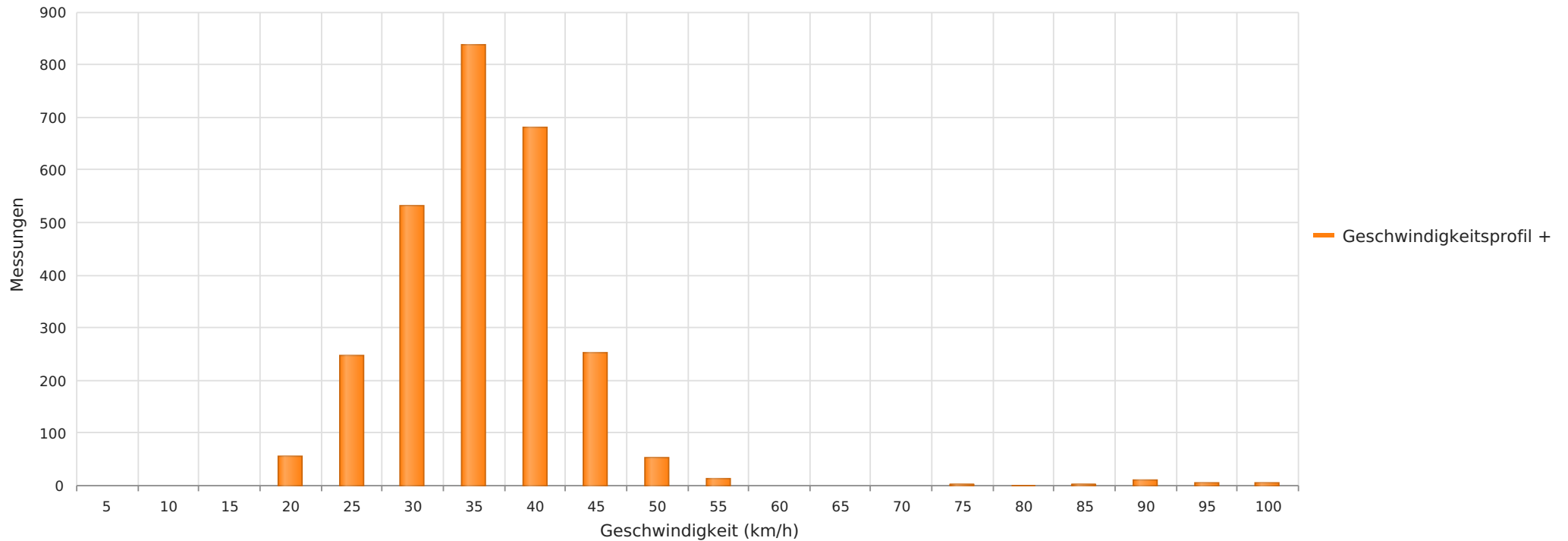
Gammen - Dorfstrasse 18B, Fahrtrichtung Biberen, 50 km/h Beschränkung Anzahl der Messwerte vs. Geschwindigkeit
