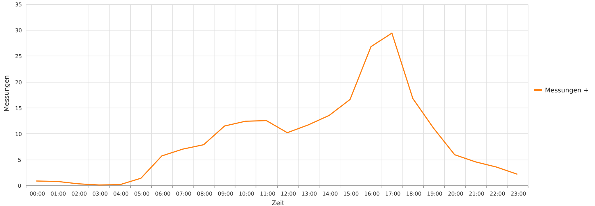
Gammen - Dorfstrasse 18B, Fahrtrichtung Biberen, 50 km/h Beschränkung Gemittelte Anzahl an Messwerten vs. Uhrzeit
